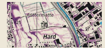
Oberflächenabflusskarte
